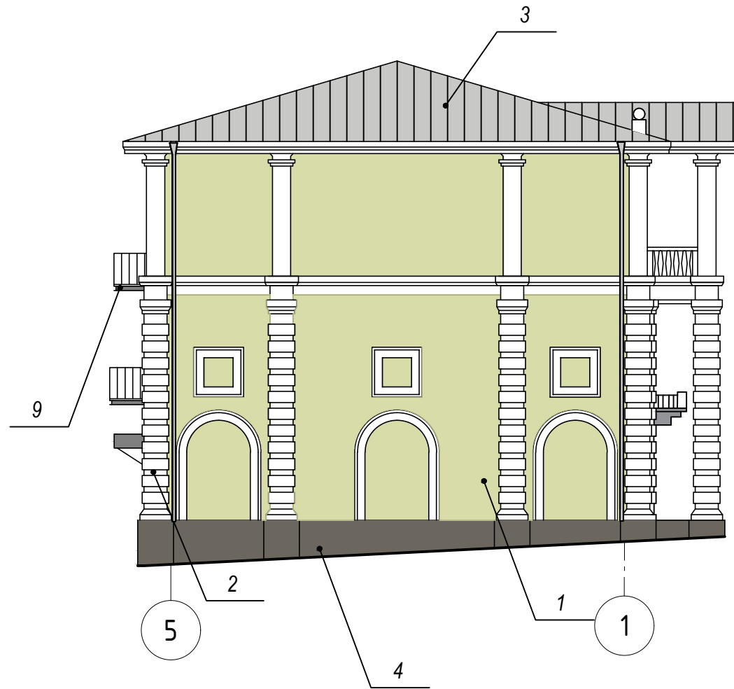
Фасад 5-1
