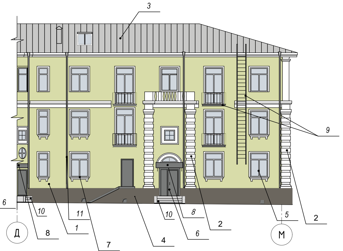
Фасад Д-М
