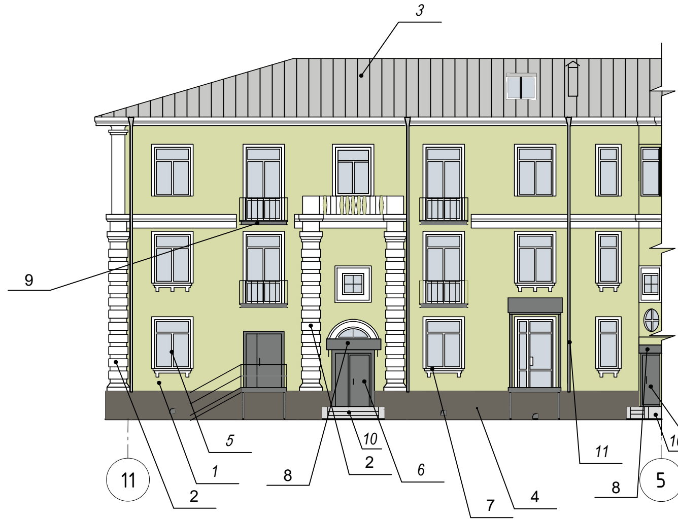
Фасад 11-5
