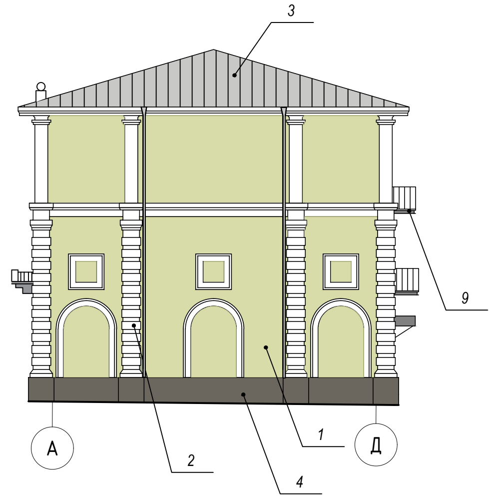
Фасад А-Д
